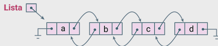
Lista duplamente encadeada.
