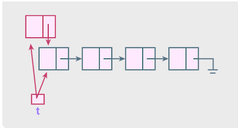
Inserção no início da lista.
